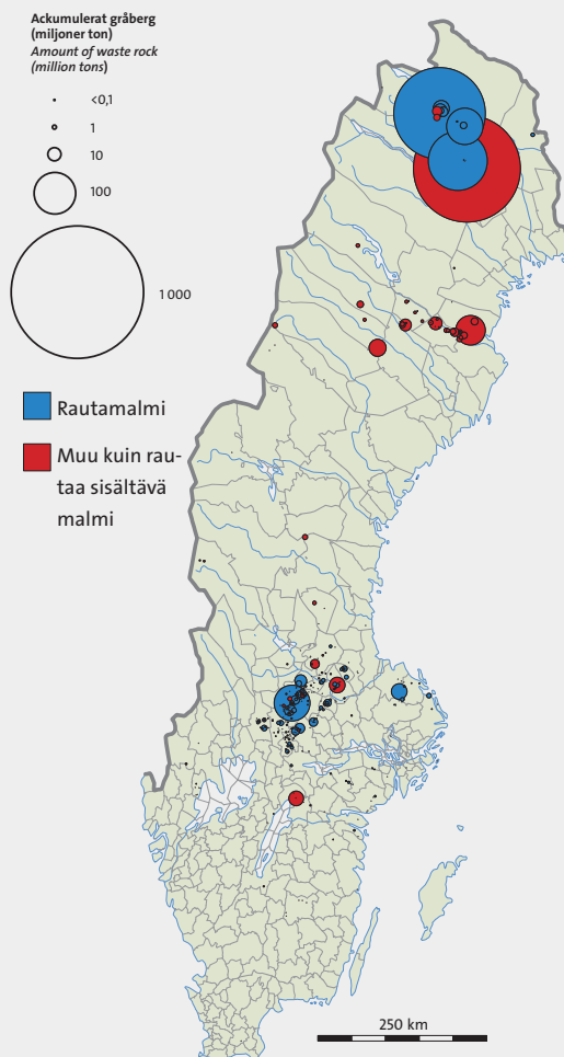
Kuva 16. Luvut SGU:n vuosittaisesta julkaisusta Bergverksstatistik 2016. Kaavio esittää tuotettua malmia, sivukiveä ja rikastushiekkaa vuositasona. Kartoissa näkyy kertynyt jäte maanlaajuisesti.
