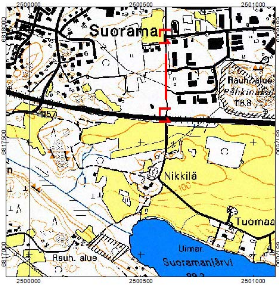
Kangasalan vastusluotauslinjan sijainti
