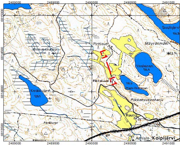
Vuoreksen vastusluotauslinjan sijainti
